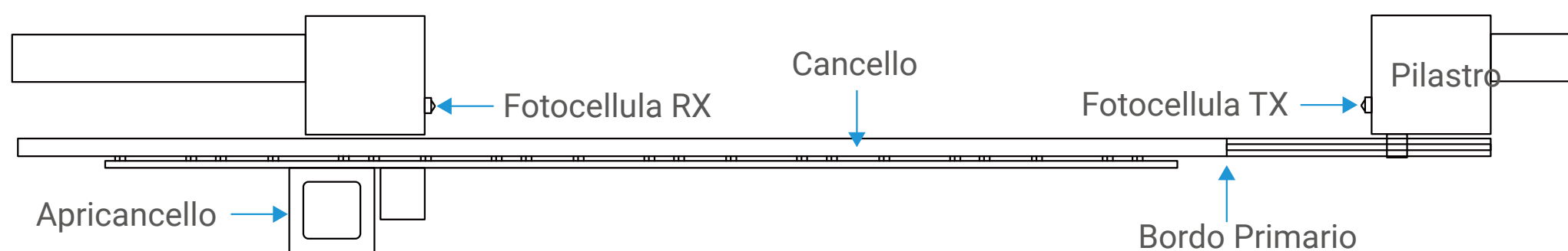
Vista dall'alto
